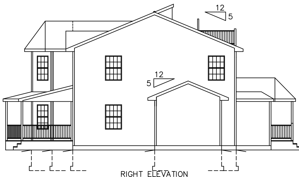
RIGHT ELEVATION
